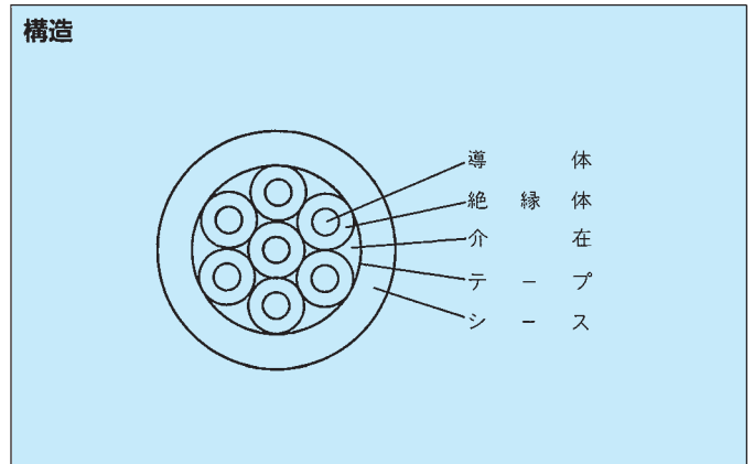
注) ケーブルグラウンドを使用する場合には、外径公差を御指示下さい。
